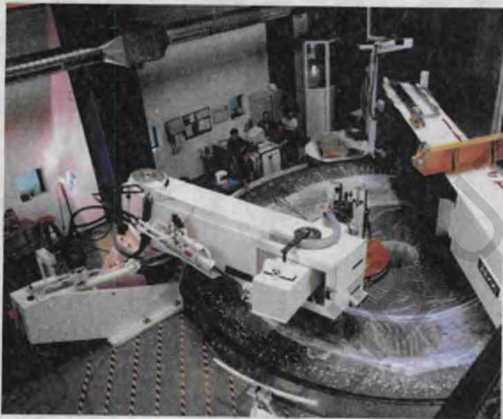
56- rasm. Diametri 8 metrli teleskop ko'zgisiga sexda sayqal berish jarayoni.
