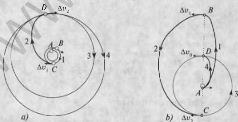
46- rasm. a) SY orbitasi balandliklarini o'zgartirish bo'yicha manyovrlar; b) ikki va uch impulsli manyovrlarni solishtirish.
