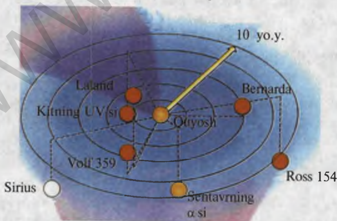
113- rasm. Quyoshdan 10 yo.y. masofagacha joylashgan yulduzlar.
