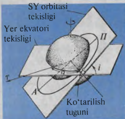
42- rasm. Yer sun'iy yo'ldoshi (YSY)ning orbita elementlari.
