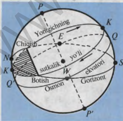
17- rasm. Yoritgichlarning kulminatsiyasi hodisasi.
