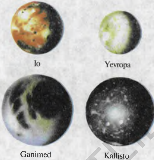
89- rasm. Yupiterning Galiley yo'ldoshlarining solishtirma o'lchamlari.
