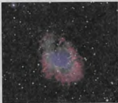
121- rasm. Savr yulduz turkumidagi Qisqichbaqasimon tumanlik – 1054- yilda portlagan o'tayangi yulduzning qoldig'i.
