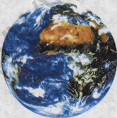
76- rasm. Yerning Oy sirtida turib olingan rasmi.
