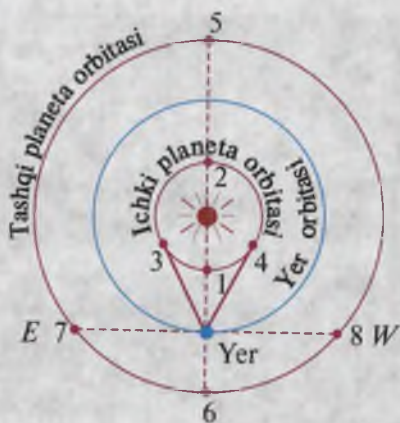
27- rasm. Planetalarning konfiguratsiyalari va ko'rinish shartlari.
