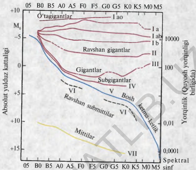
111- rasm. Yulduzlarning yorqinlik sinflari.
