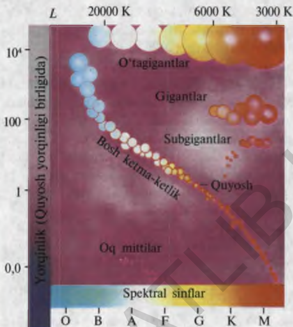
110- rasm. Spektr-yorqinlik diagrammasi.
