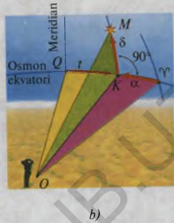
13- rasm. Ekvatorial koordinatalar sistemalari.
