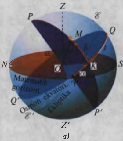
13- rasm. Ekvatorial koordinatalar sistemalari.
