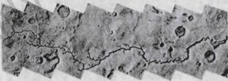
83- rasm. Marsning Nirgal deb nom olgan daryo o‘zani (uzunligi 400 km dan ortiq).
