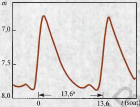
119- rasm. Liraning RR o'zgaruvchi yulduzi ravshanligining o'zgarishi.
