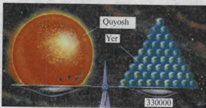
25- rasm. Yer massasini Quyosh massasi bilan solishtirish.
