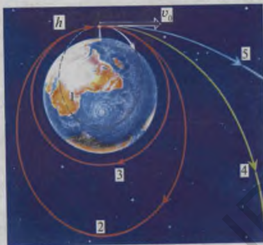
39- rasm. Tortishishning markaziy maydonida jismning harakat trayektoriyalari (misol tariqasida, Yer tortishish maydonida KA ning harakati keltirilgan).
