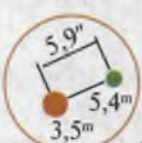
Gerkulesning \alpha si
