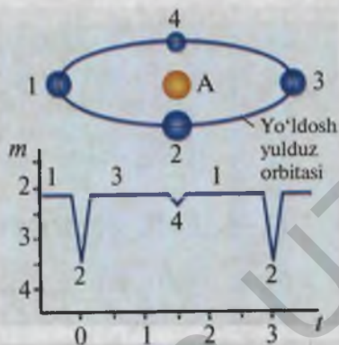
117- rasm. Tutiluvchi qo'shaloq yulduz:
