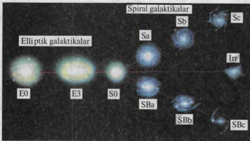
135- rasm. Galaktikalarning evolutsiyasi.
