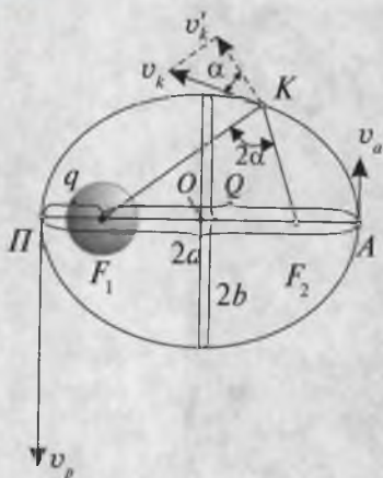
40- rasm. Tortishishning markaziy maydonida jismining elliptik trayektoriya bo'ylab harakati.
