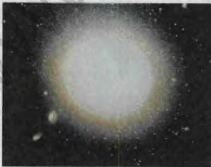
133- rasm. Elliptik galaktika.
