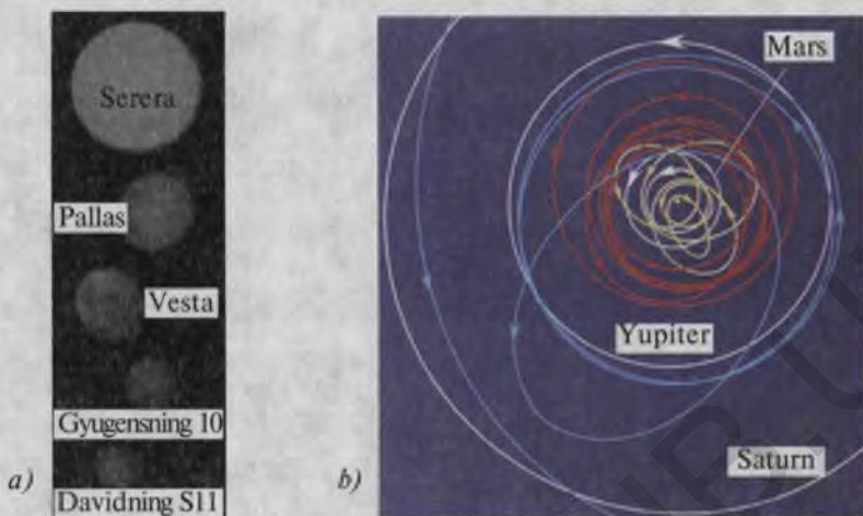
100- rasm. a) taniqli mayda planetalarning solishtirma o'lchamlari (M 1 sm : 500 km); b) bir guruh mayda planetalarning orbitalari.
