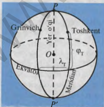
12- rasm. Geografik koordinatalar sistemasi.
