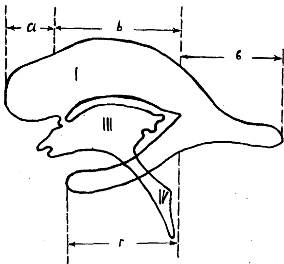
10- расм. Мия қоринчалари ён тасвирининг тузилиши: а — олдинги шоҳча; б — тана шоҳча; в — орқа шоҳча; г — пастки шоҳча.
