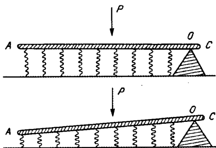
3.28-расм. Ёйсимон протез чекка эгарининг юкланиш схемаси:
