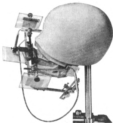
4.28-расм. Сагиттал бўғимли, сагиттал кесиш ва трансверзал кесиш йўлларининг оғиздан ташқаридаги ёзувини ҳосил қилиш учун бош фантомига ўрнатилган юз ёйи.
